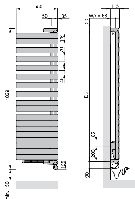
Elektrobetrieb: Ausführung links
